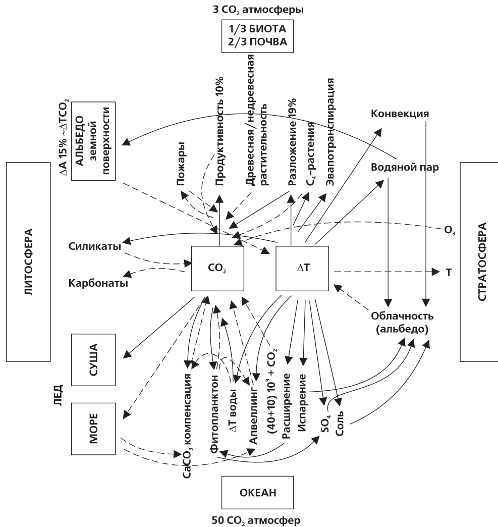
Рис. 4. Схема регуляции содержания атмосферной CO 2 . (Красилов, 1992.)
