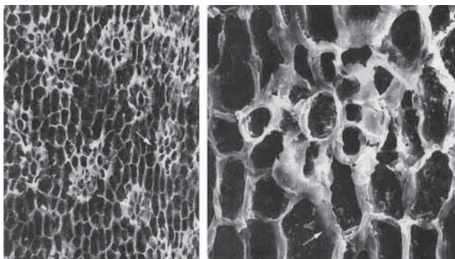
Рис. 2. Полиморфизм устьичных аппаратов у пермского хвойного Ullmannia cf. bronnii Goepfert. Абортированный устьичный аппарат (стрелка) в виде скопления мелких мезогенных клеток, образующих в зрелом мезоперигенном аппарате (справа) кольцо побочных клеток, прерванное вклинивающейся перигенной клеткой. (Красилов, 2004.)
