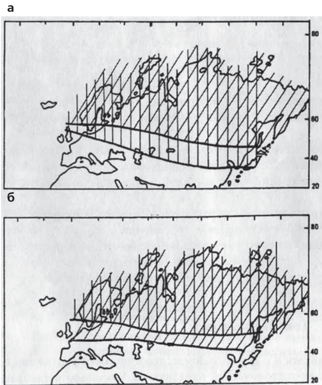
Рис. 3. Положение границы субтропической и умеренной (заштрихована) фитоклиматических областей в средней юре — раннем мелу (а) и позднем мелу — палеогене (б).
