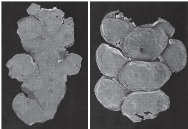
Рис. 1. Полиморфизм переходных форм от чешуелистных побегов к филлокладиям у голосеменного растения из пермских отложений Европейской России. (Карасев, Красилов, 2008.)
