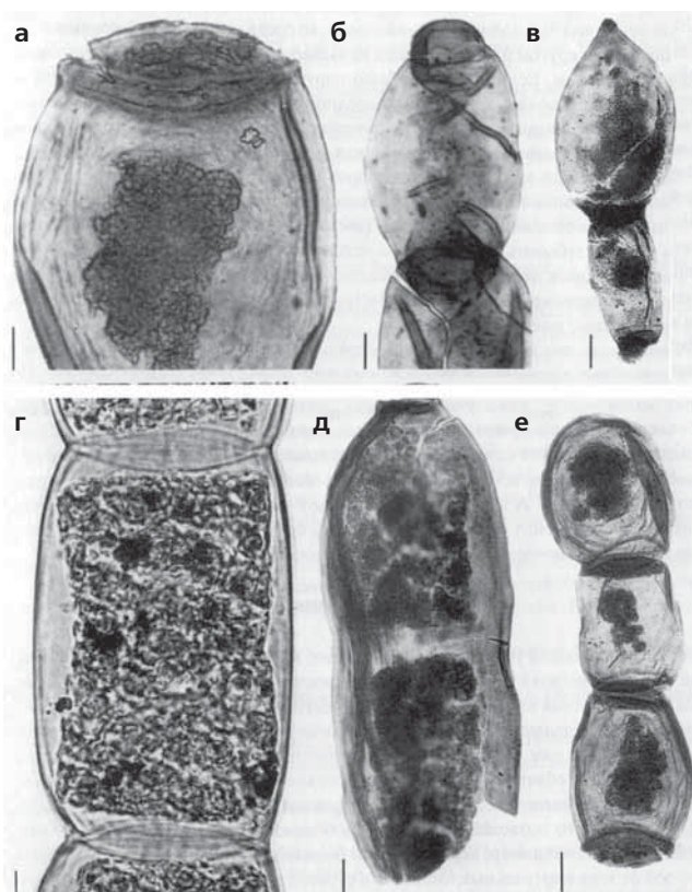
Рис. 5. Tumulicysta из пограничных отложений перми и триаса Русской платформы. Колонии вегетативных клеток и акинеты (слева внизу для сравнения фрагмент нитчатой колонии современной водоросли Spirogyra sp. ). Длина масштабной линейки: а, б, г, д — 10 мкм; в — 20 мкм; е — 30 мкм.
